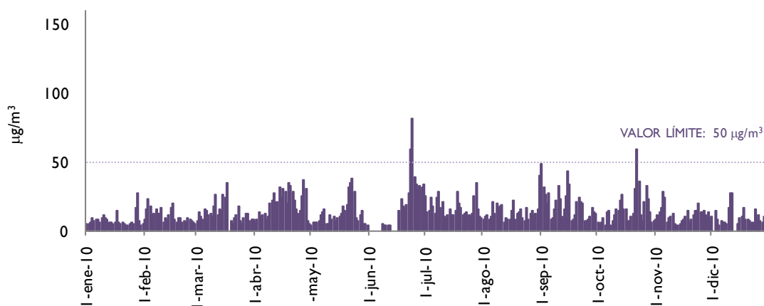
Figura 17/ PM_{10} : Evolución de valores diarios en Santa Margarita (2010. Datos corregidos)
