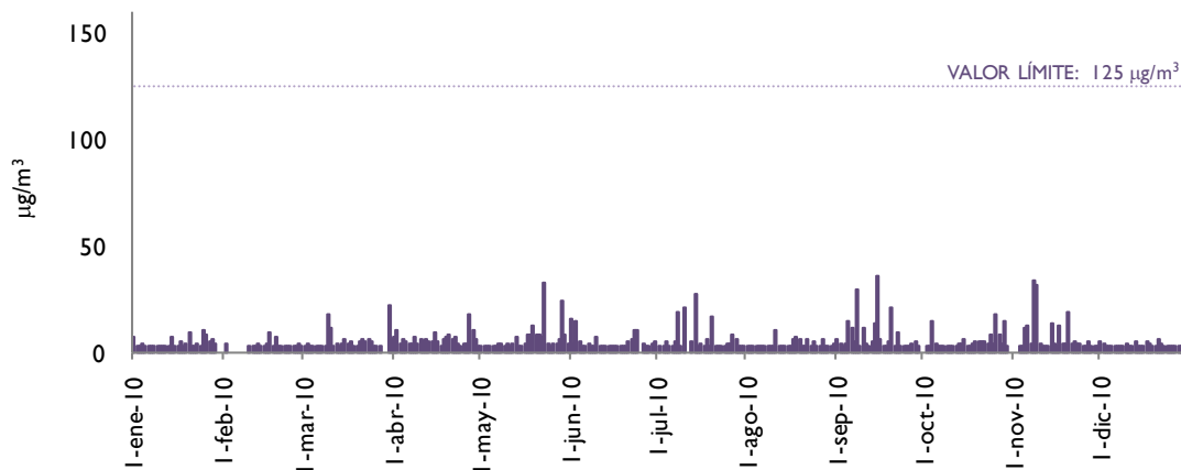
Figura 7/ SO 2 : Evolución de valores diarios en Pablo Iglesias (2010)
