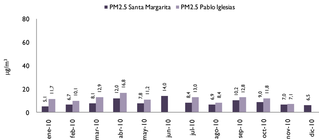
Figura 33/ PM 2.5 : Evolución de valores mensuales (Valores sin corregir. 2010)
