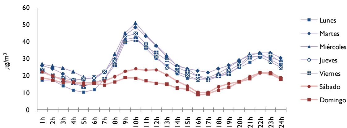
Figura 14/ \text{NO}_2 : Perfil diario de promedios horarios (Santa Margarita, 2010)
