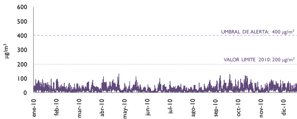
Figura 9/ NO 2 : Evolución de valores horarios en Santa Margarita (2010)
