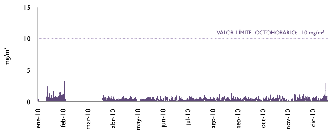
Figura 27/ Monóxido de Carbono: Evolución de valores horarios en Santa Margarita (2010)
