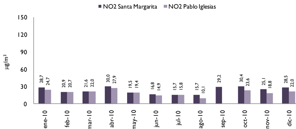
Figura 30/ Dióxido de Nitrógeno: Evolución de valores mensuales (2010)
