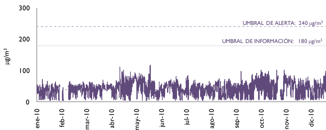
Figura 23/ Ozono: Evolución de valores horarios en Pablo Iglesias (2010)
