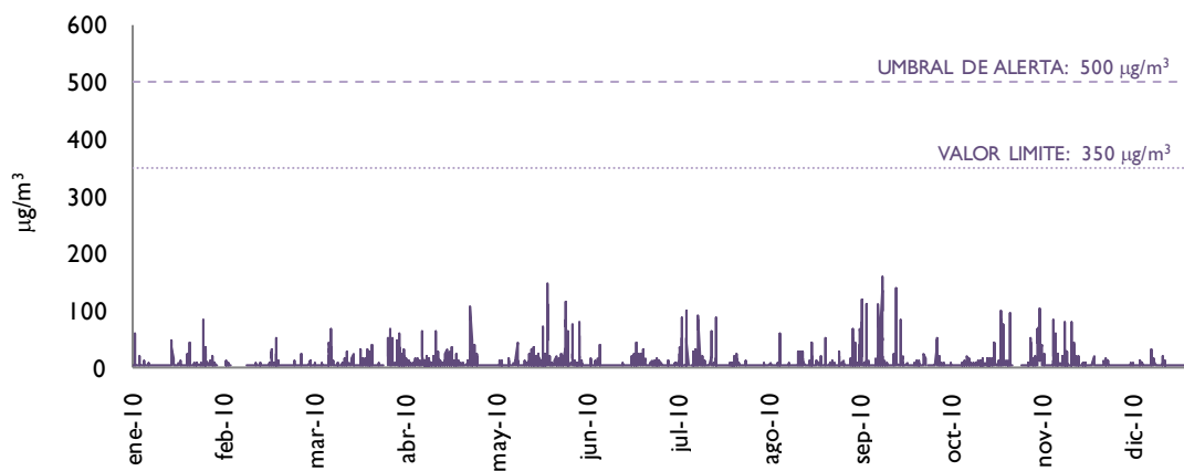
Figura 5/ SO 2 : Evolución de valores horarios en Pablo Iglesias (2010)
