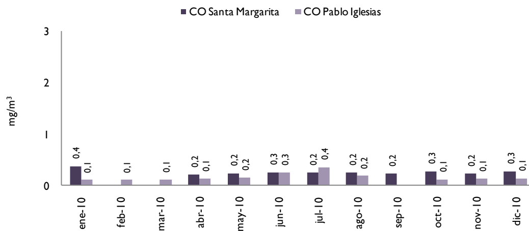
Figura 35/ Monóxido de Carbono: Evolución de valores mensuales (2010)
