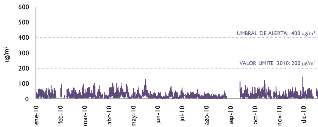
Figura 10/ NO 2 : Evolución de valores horarios en Pablo Iglesias (2010)
