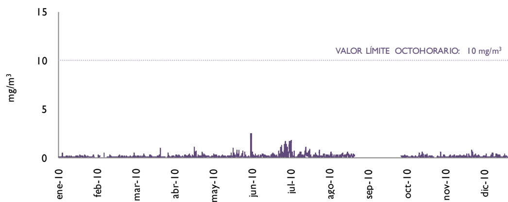
Figura 28/ Monóxido de Carbono: Evolución de valores horarios en Pablo Iglesias (2010)
