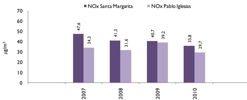
Figura 12/ NO x : Evolución de valores anuales
