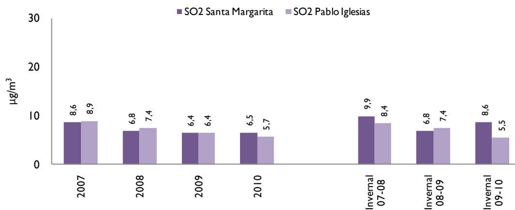
Figura 8/ SO 2 : Evolución de valores anuales e invernais
