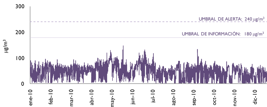
Figura 22/ Ozono: Evolución de valores horarios en Santa Margarita (2010)
