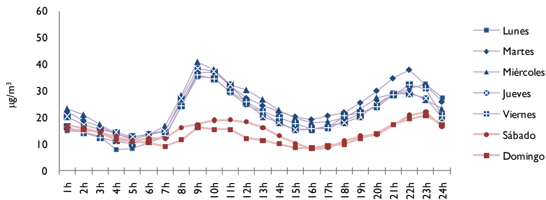
Figura 15/ NO 2 : Perfil diario de promedios horarios (Pablo Iglesias, 2010)
