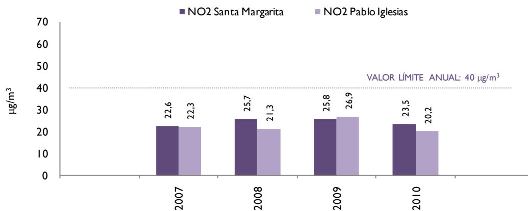
Figura 11/ NO 2 : Evolución de valores anuales
