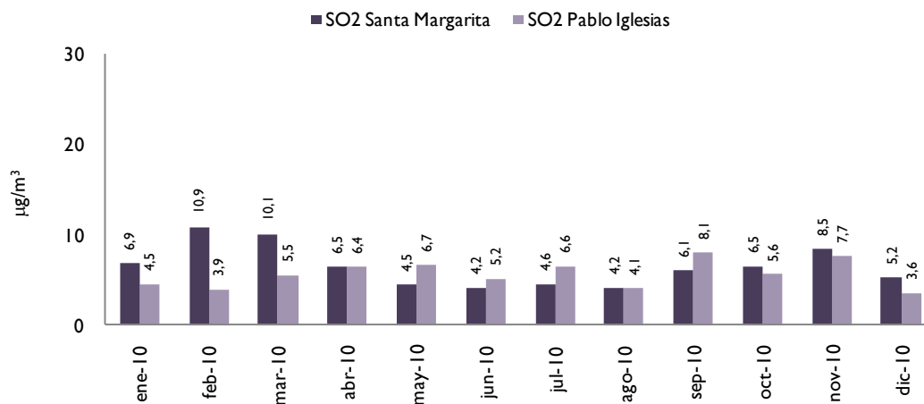
Figura 29/ Dióxido de Azufre: Evolución de valores mensuales (2010)
