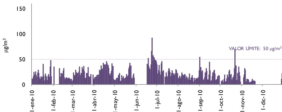
Figura 18/ PM 10 : Evolución de valores diarios en Pablo Iglesias (2010. Datos corregidos)
