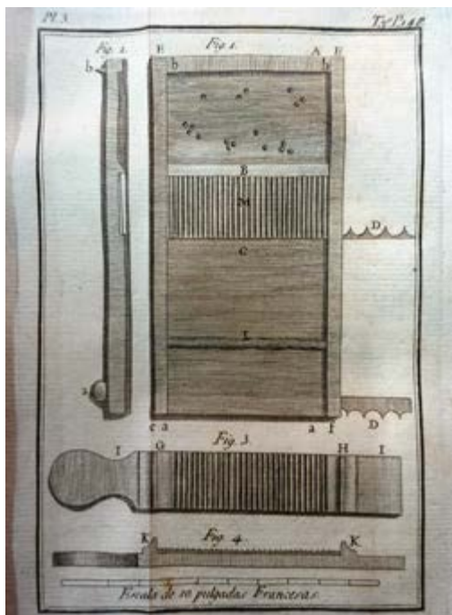
Estampa máquina alemana para dividir y redondear píldoras, 1793. 147
