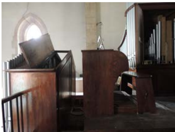
San Francisco. Vista lateral. Cadereta aberta, consola superior e corpo principal aberto.
