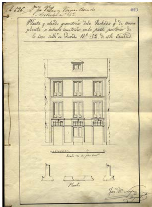
Plano de planta y alzado geométrico de la fachada en parte posterior de casa n.º 52 de c/Acevedo, 1853 125 . [Farmacia Villar].
